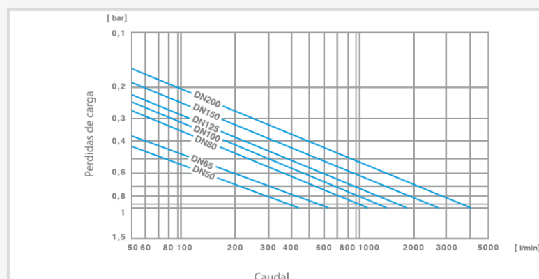
DIAGRAMA DE CAUDALES Y PÉRDIDAS DE CARGA
